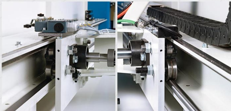
Movimentazione con pignoni e cremagliere e posizionamento tramite sensore e banda magnetica Movement and positioning by racks and pinions with sensor and magnetic strip Desplazamiento y posicionamiento con cremalleras y piñones de movimiento a través de sensor y banda magnética Bewegung mit Ritzel und Zahnstangen und Positionierung durch Sensor und Magnetband Mouvement et positionnement avec pignon et crémaillère au moyen du capteur et bande magnétique
